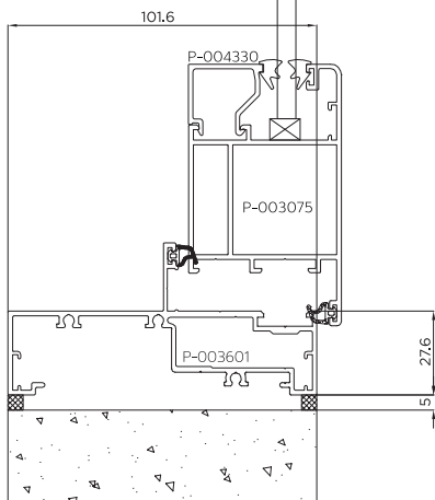
เฟรมบน-ล่าง หน้าต่าง ขนาด 4"
