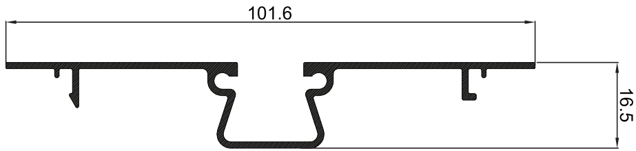
P-003093 ตบร่องยาว ER
