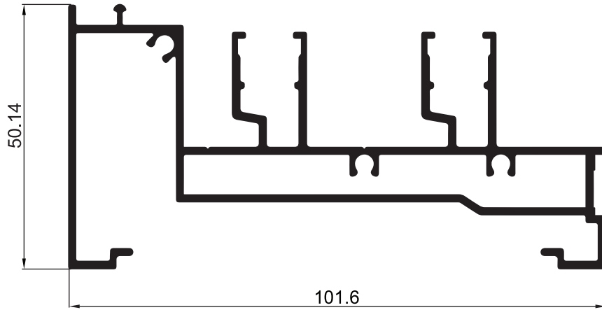
P-124563 / 154465 เฟรมบน-ล่างบานเลื่อน 4" ( 2 ราง )
