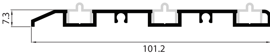
P-154309 เฟรมล่างภายใน 3 ราง
