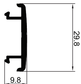
P-003042 ฝาปิดเสาเสริมความแข็งแรง
