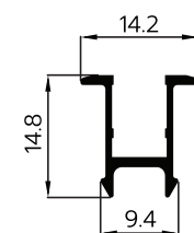
NEW P-084963 Adapter รางสแตนเลส
