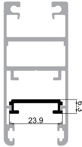
P-007227 ซีเสริมบาน ER
