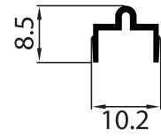
P-104311 รางล้อยภายใน
