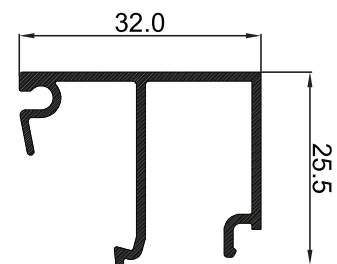
G-006061 คิ้วเหลี่ยม ER
