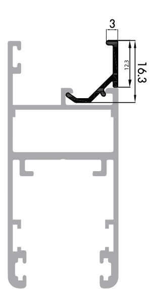
P-123119 คิ้ว (กระจก 20 มม.) ยางอัด-ยางวางกระจก
