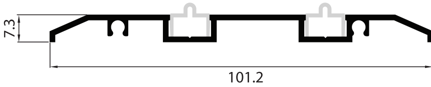
P-154310 เฟรมล่างภายใน 2 ราง
