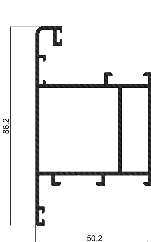
P-003075 กรอบบานเปิด ER 4" ยางลูกโป่งฐาน 4.8x6.5 มม. ยางฉัด-ยางวางกระจก
