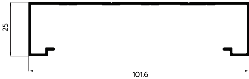
NEW P-124941 / 154942 เฟรมข้างบานเลื่อน
