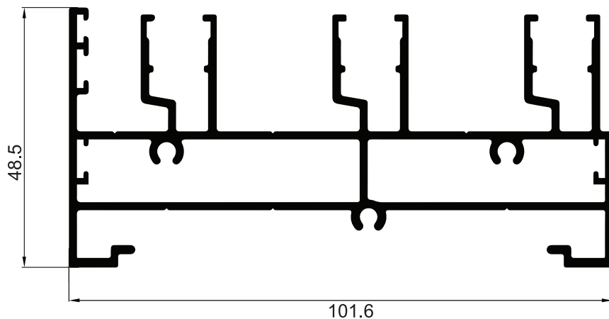
P-124562 / 154307 เฟรมบานเลื่อน 4" ( 3 ราง ) ร่องลึกหลายฐาน 5x5 มม.
