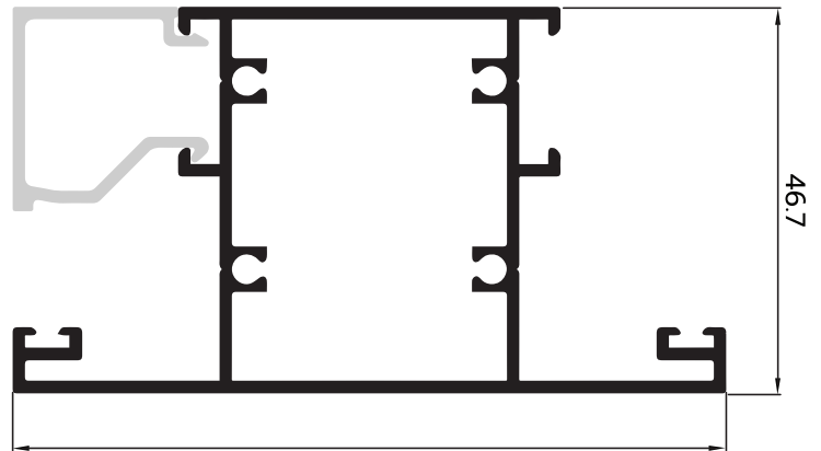
NEW P-154516 แม่ทงกระจก 4" ยางอัด-ยางวางกระจก
