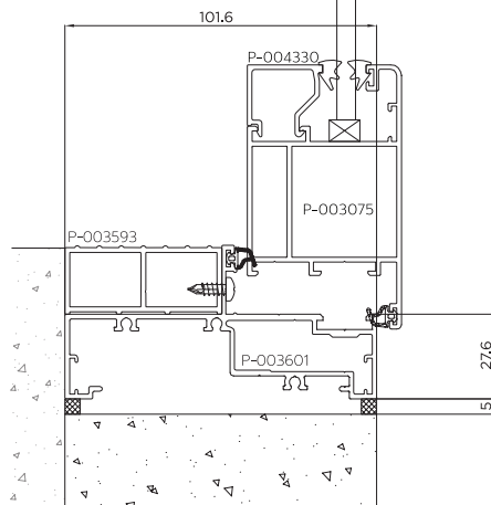
เฟรมล่างประตู ขนาด 4"
