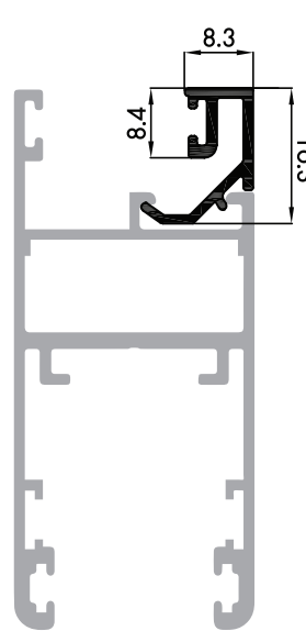
P-123118 คิ้ว (กระจก 10 มม.) ยางอัด-ยางวางกระจก
