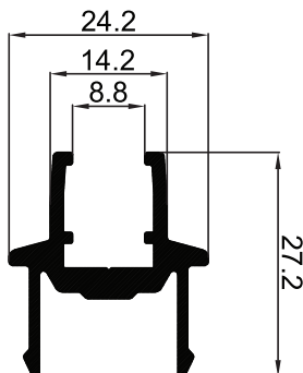
P-009414 ซนกลางบานเลื่อน
