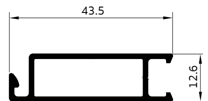
2006 กรอบมุ้ง บานเลื่อน
