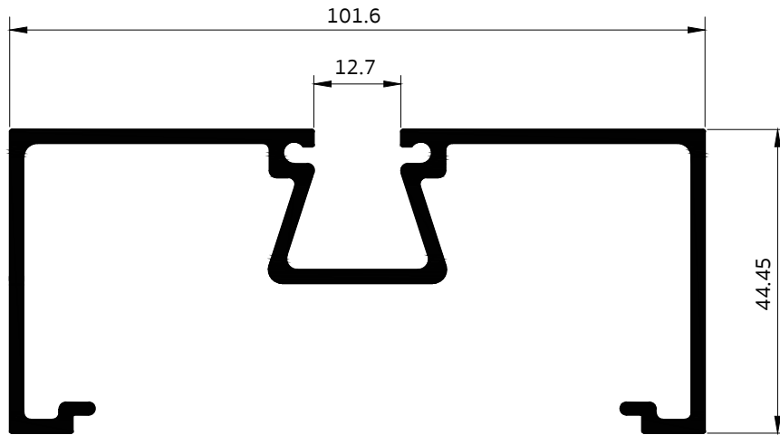
3012 กล่องร่อง 4"
