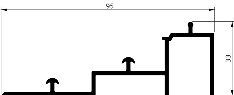
4112 เฟรมล่างชั้นบันได
