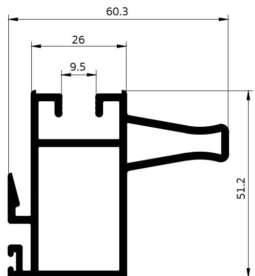
14091 เสาก๊วยมือจับ 2"
