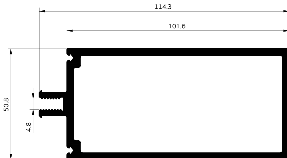
230009 เสาเคอร์วอลส์ 2" x 4"
