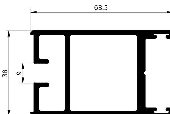
4054 เสาฤดูแฉงตัวเมียบ น๊ิกเฟรม
