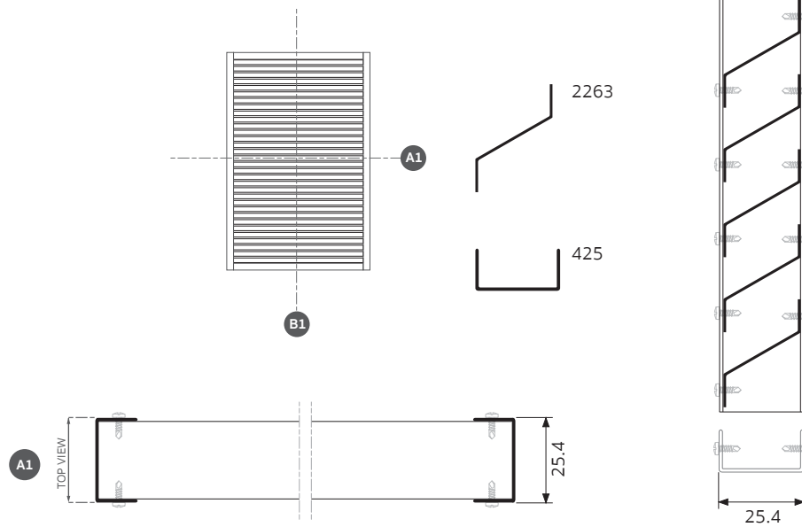
ระแนงบังแดด เหล็ก Z กว้าง 1"
