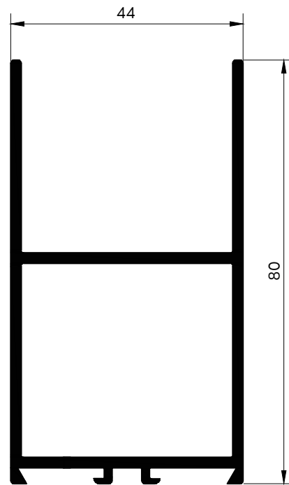
3032 ขวางล่างประตูสวิตช์
