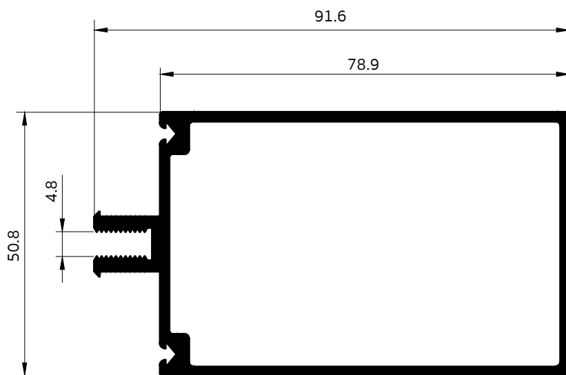
19013 เสาเคอร์วอลส์ 2" x 3"
