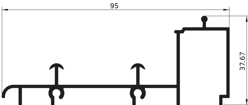
4394 เฟรมล่างขาสูง (ไม่มีฉากกันตก)
