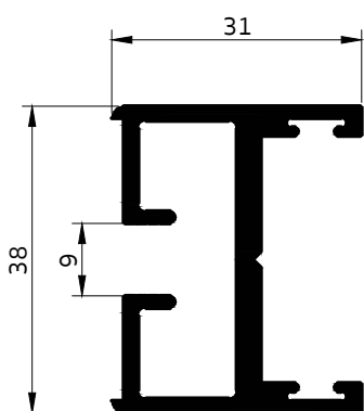
4057 เสาดาย น๊ิกเฟรม
