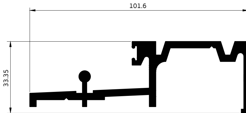
4055 เฟรมล่างน๊ิกเฟรม
