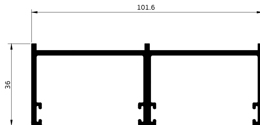
4056 เฟรมบนน๊ิกเฟรม
