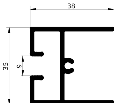
4060 ขวางบน น๊ิกเฟรม
