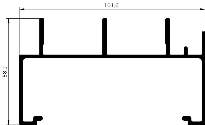
4870 เฟรมบน ติดกล่อง 4"
