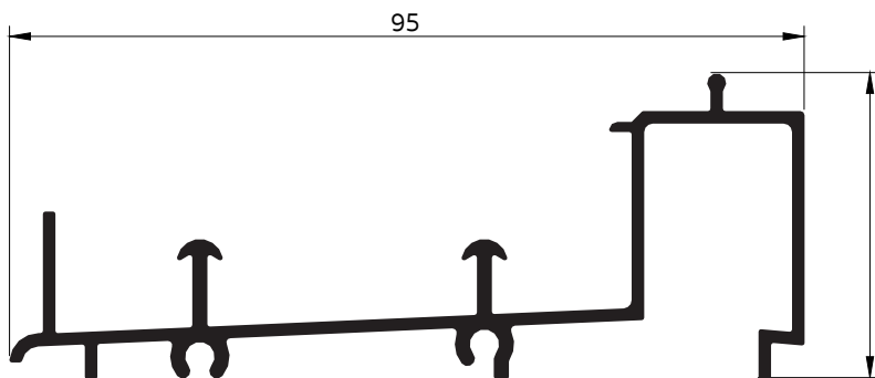
4800 เฟรมล่างขาสูง (มีฉากกันตก)
