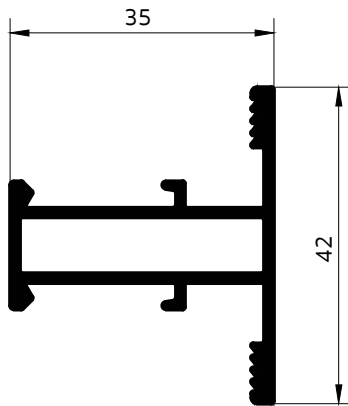
5009 ชอยกลางบานกระทุ้ง
