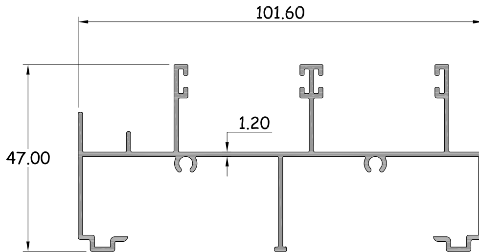
เฟรมบน รหัสสินค้า : 15100 WT. 0.992 Kg / M.
