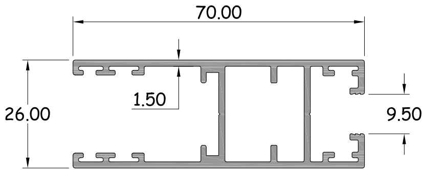
กรอบบานเลื่อน 70 มิล รหัสสินค้า : 15146 WT. 1.028 Kg / M.
