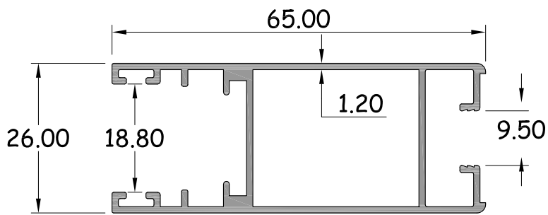
เสาเกี่ยว+เสาถูกแฉ รหัสสินค้า : 15105 WT. 0.704 Kg / M.
