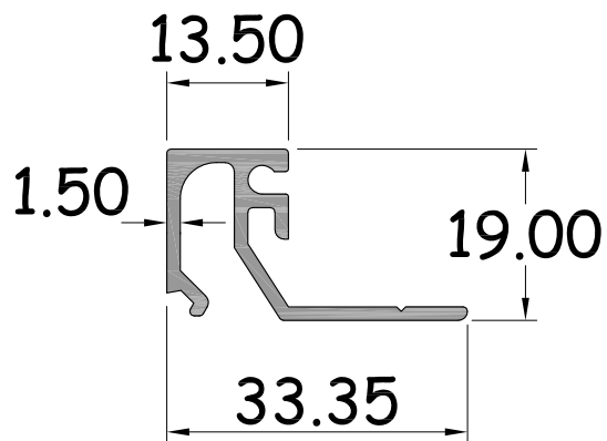
คิ้วนอกบานเพิ่มร่องกระจก 25.0 มิล รหัสสินค้า : 15175 WT. 0.340 Kg / M.
