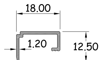
กรอบมุ้งนिरภัย รหัสสินค้า : 15132 WT. 0.717 Kg / M.
