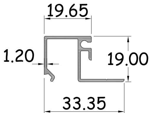
คิ้วนอกบานเพิ่มหนา 1.20 มิล รหัสสินค้า : 15185 WT. 0.266 Kg / M.
