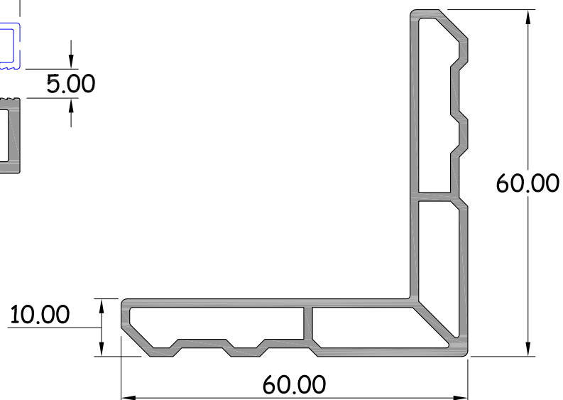
ฉากเข้ามุม บานเลื่อน EURO หนา 1.5 มิล รหัสสินค้า : 15152 WT. 1.035 Kg / M.
