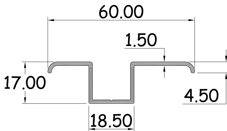
เฟรมล่างภายในบานเพี้ยม รหัสสินค้า : 15170 WT. 0.380 Kg / M.
