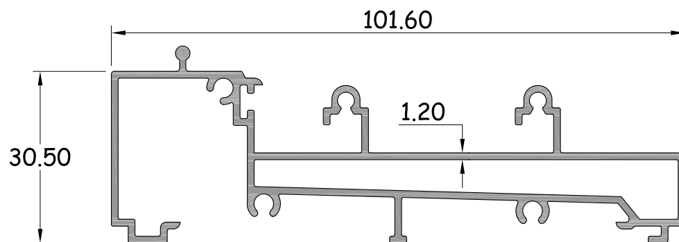
เฟรมล่าง (HOLLOW) รหัสสินค้า : 15134 WT. 1.153 Kg / M.
