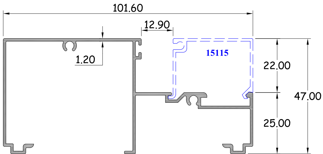
วงกบไม้ รหัสสินค้า : 15121 WT. 0.874 Kg / M.
