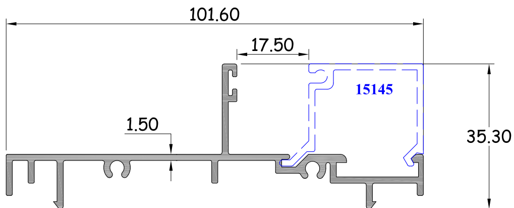
คาน C กรูฟ หนา 1.5 มิล รหัสสินค้า : 15160 WT. 0.848 Kg / M.
