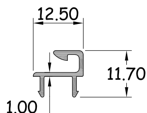
ตบเกี้ยว 2 ทาง รหัสสินค้า : 15128 WT. 0.459 Kg / M.
