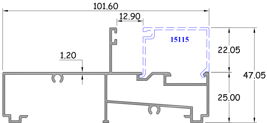
กล่องก้าน (HOLLOW) รหัสสินค้า : 15131 WT. 0.938 Kg / M.
