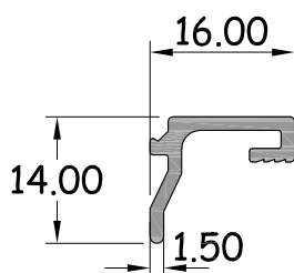
คิ้วตบกรอบบานเลื่อน หน้า 1.5 มิล รหัสสินค้า : 15148 WT. 0.148 Kg / M.
