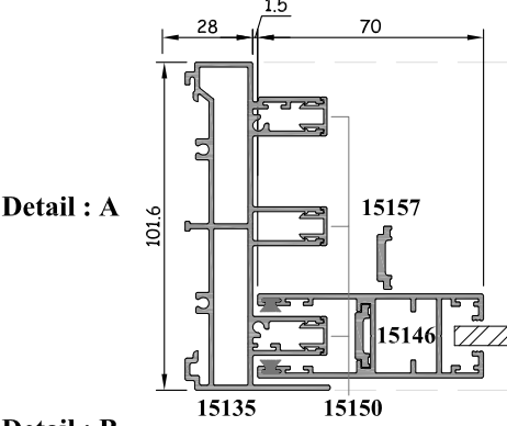
กรณีใช้เฟรม 15135
