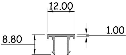
คานาข้าง รหัสสินค้า : 15150 WT. 0.074 Kg / M.
