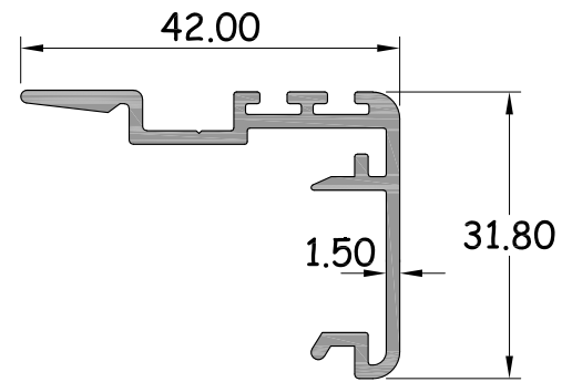
ตบเกี่ยวหนา 1.5 มิล รหัสสินค้า : 15158 WT. 0.468 Kg / M.
