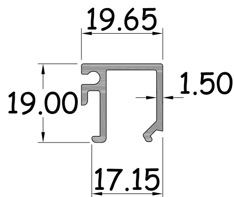
คิ้วในบานเพ็ญร่องกระบอก 12.7 มิล รหัสสินค้า : 15174 WT. 0.280 Kg / M.
