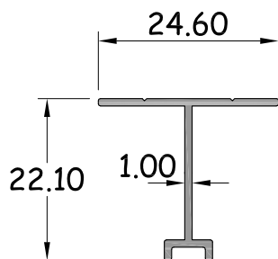
อแดปเตอร์ต่อเฟรม EURO รหัสสินค้า : 15191 WT. 0.143 Kg / M.
