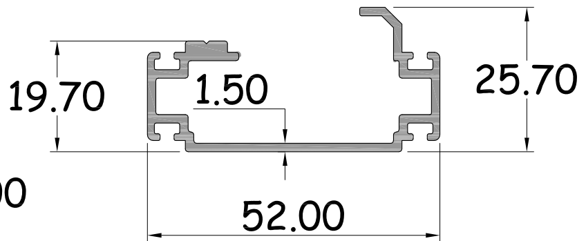
แกนกลางบานเพ็ญ รหัสสินค้า : 15178 WT. 0.592 Kg / M.
