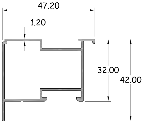
บังใบบานเปิดคู่ รหัสสินค้า : 15124 WT. 0.534 Kg / M.
