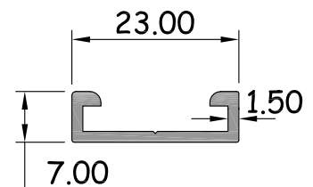
เส้นเสริม C กรูฟ หน้า 1.5 มิล รหัสสินค้า : 15179 WT. 0.162 Kg / M.
