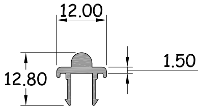
คานาเลื่อน รหัสสินค้า : 15149 WT. 0.130 Kg / M.
