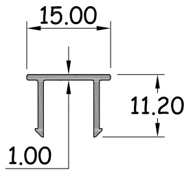
ฝาปิดเดือยกุญแจ รหัสสินค้า : 15112 WT. 0.094 Kg / M.
