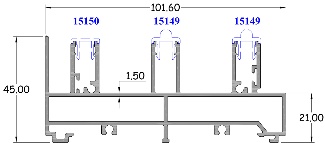
เฟรม 3 ร่อง HOLLOW รหัสสินค้า : 15135 WT. 1.958 Kg / M.
