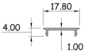
ตบปิดกล่องกัน รหัสสินค้า : 15156 WT. 0.058 Kg / M.
