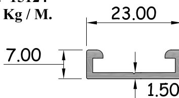
เส้นเสริม C กรูฟ หนา 1.5 มิด รหัสสินค้า : 15179 WT. 0.162 Kg / M.
