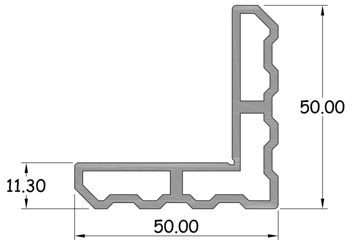
ฉากเข้ามม บานเปิดกรอบ 65 มิด C กรูฟ รหัสสินค้า : 15188 WT. 1.142 Kg / M.
