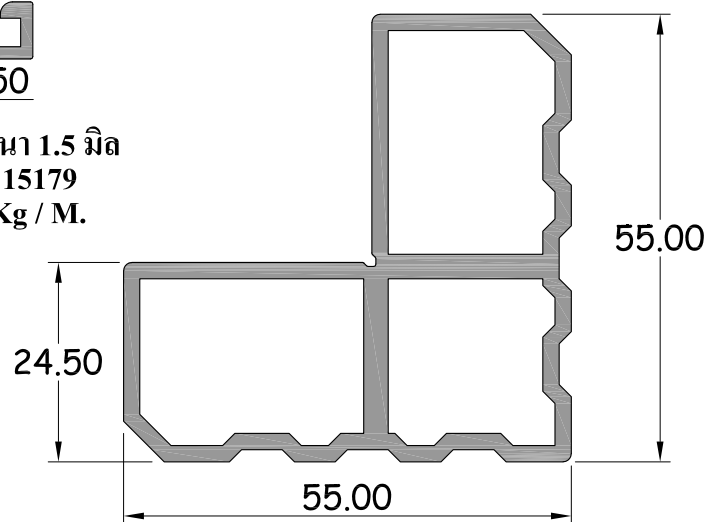
ฉากเข้ามม บานเปิดกรอบ 80 มิด รหัสสินค้า : 15189 WT. 1.465 Kg / M.
