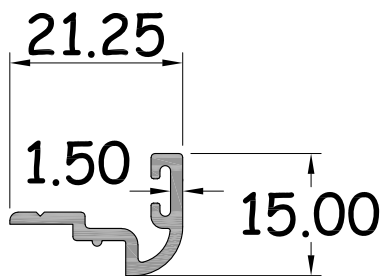
บังใบบานเพ็ญ รหัสสินค้า : 15177 WT. 0.184 Kg / M.
