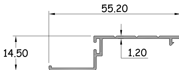
ตบรู้น้ำเตี้ย รหัสสินค้า : 15107 WT. 0.227 Kg / M.
