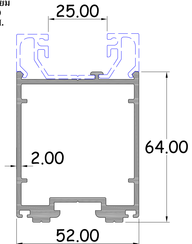
เสาบานเพี้ยม หน้า 2.0 มัด รหัสสินค้า : 15172 WT. 1.592 Kg / M.
