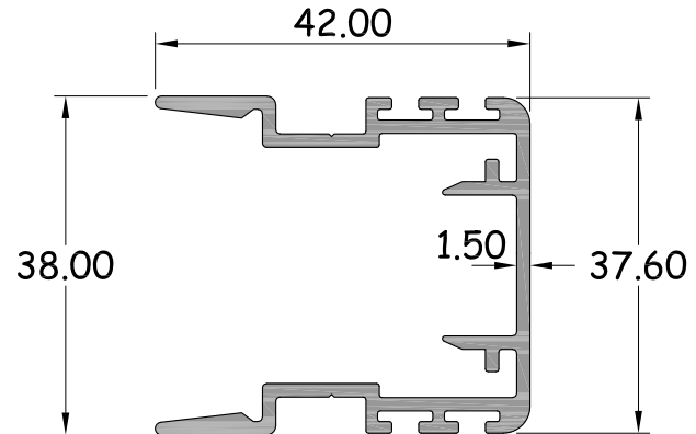
ตบเกี่ยว 2 ทาง หนา 1.5 มิล รหัสสินค้า : 15159 WT. 0.729 Kg / M.
