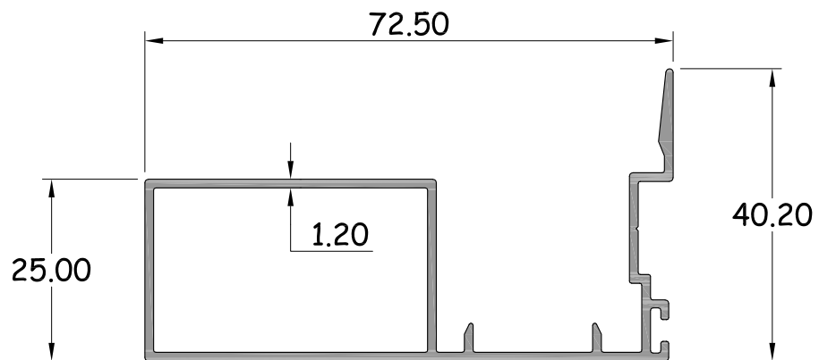
ตบเกี้ยวโหนก รหัสสินค้า : 15130 WT. 0.706 Kg / M.
