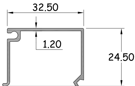
ก๊วยตบกระจก รหัสสินค้า : 15115 WT. 0.267 Kg / M.
