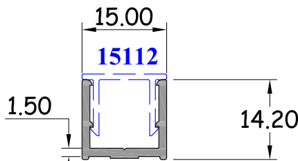
เดือยกุญแจ หน้า 1.5 มิล รหัสสินค้า : 15183 WT. 0.163 Kg / M.
