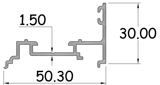
แกนกลางบังใบบานเพ็ญ V2 / บังใบเข้ามุม 90 รหัสสินค้า : 15196 WT. 0.505 Kg / M.
