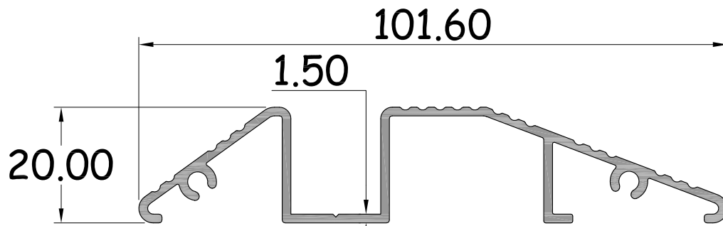
เฟรมล่างหลังเต่าบานเพี้ยม รหัสสินค้า : 15194 WT. 0.739 Kg / M.
