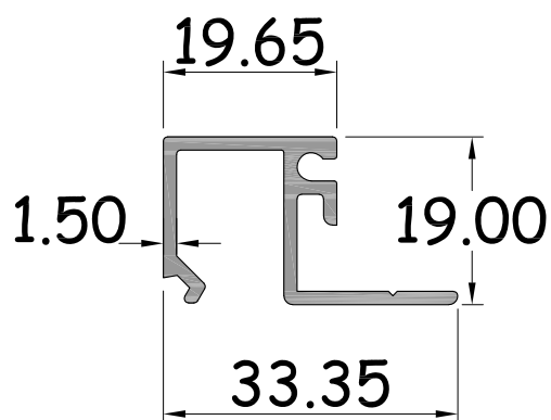
คิ้วนอกบานเพ็ญร่องกระบอก 12.7 มิล รหัสสินค้า : 15173 WT. 0.345 Kg / M.
