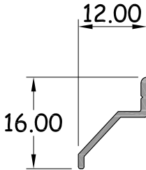
ใบบังฝน รหัสสินค้า : 15138 WT. 0.061 Kg / M.
