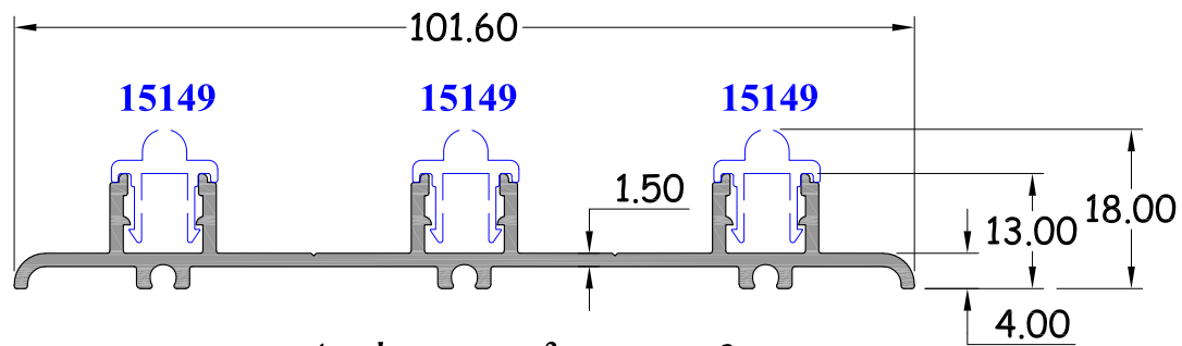
เฟรมล่าง 3 รางภายใน หน้า 1.5 มิล รหัสสินค้า : 15184 WT. 0.720 Kg / M.
