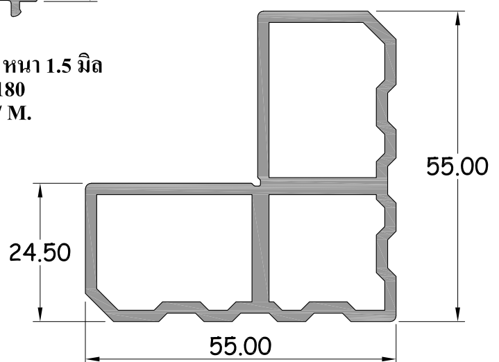
ฉากเข้ามุม บานเปิดกรอบ 80 มิล รหัสสินค้า : 15189 WT. 1.465 Kg / M.
