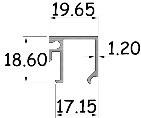
คิ้วในบานเพิ่มหนา 1.20 มิล รหัสสินค้า : 15186 WT. 0.217 Kg / M.
