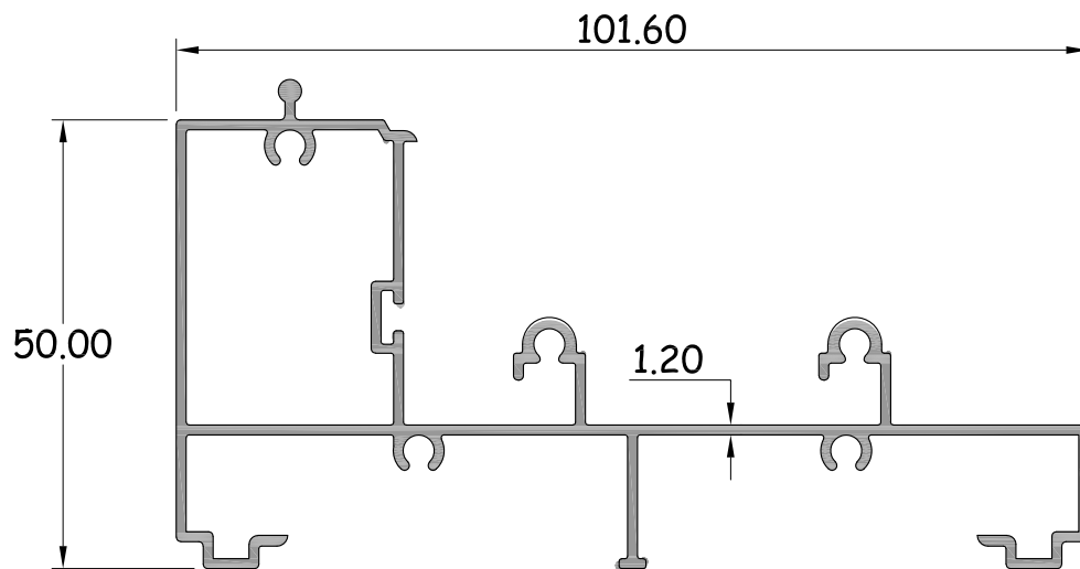
เฟรมล่างขาสูง รหัสสินค้า : 15103 WT. 1.000 Kg / M.
