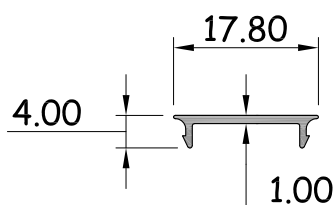
ดบปิดกล่องกัน รหัสสินค้า : 15156 WT. 0.058 Kg / M.
