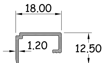
คานาครอบมุ้งนิกาย รหัสสินค้า : 15133 WT. 0.117 Kg / M.
