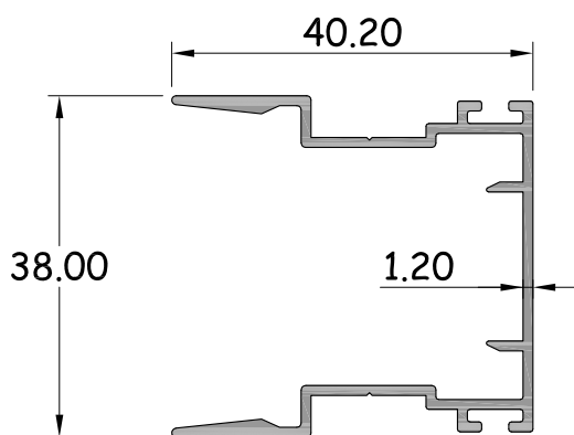
ตบเกี้ยว 2 ทาง รหัสสินค้า : 15128 WT. 0.459 Kg / M.
