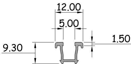
คานารับแท่งสแตนเลส รหัสสินค้า : 15161 WT. 0.083 Kg / M.
