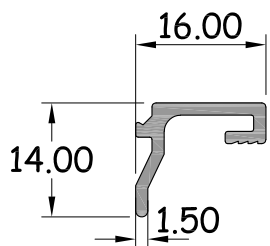
คานาครอบบานเลื่อน หน้า 1.5 มิล รหัสสินค้า : 15148 WT. 0.148 Kg / M.
