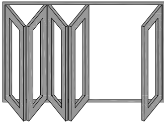
เพี้ยม 5-4-1
