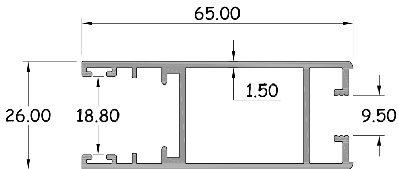
เสาเกี่ยว+เสาถูกแฉ หน้า 1.5 mm. รหัสสินค้า : 15136 WT. 0.891 Kg / M.
