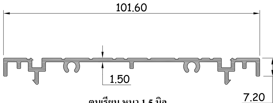
ดบเรียบ หน้า 1.5 มิล รหัสสินค้า : 15164 WT. 0.656 Kg / M.
