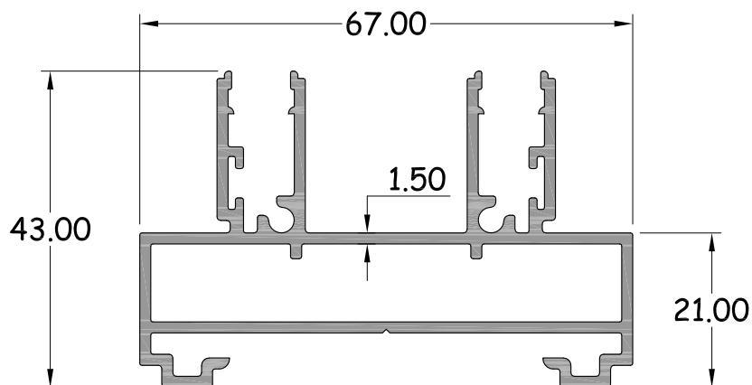
เฟรม 2 ราง HOLLOW รหัสสินค้า : 15190 WT. 1.279 Kg / M.
