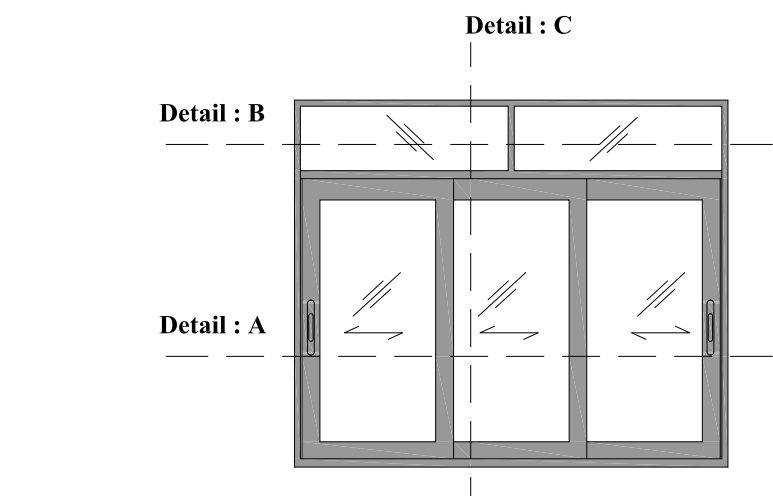
กรณีประกอบเฟรม 45 °
