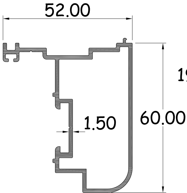
เสาบานเพ็ญเข้ามุม 90 รหัสสินค้า : 15195 WT. 0.931 Kg / M.
