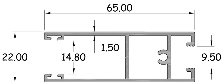
ขวางบน+ขวางล่าง หน้า 1.5 mm. รหัสสินค้า : 15137 WT. 0.816 Kg / M.
