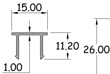
ฝาปิดเดือยกุกญแ รหัสสินค้า : 15112 WT. 0.094 Kg / M.
