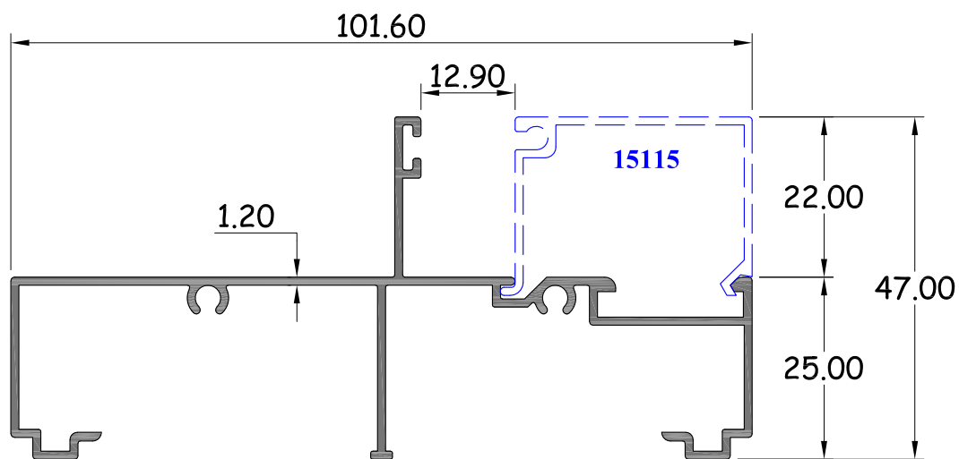
กล่องก้าน C กรูฟ รหัสสินค้า : 15200 WT. 0.795 Kg / M.
