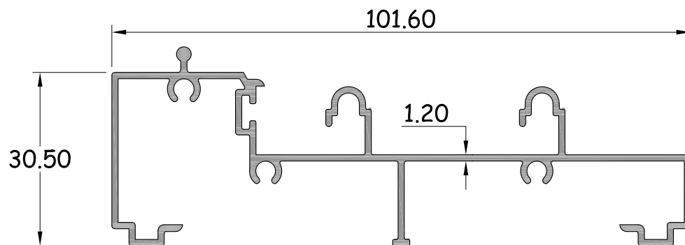
เฟรมล่างขาเดียว รหัสสินค้า : 15101 WT. 0.869 Kg / M.
