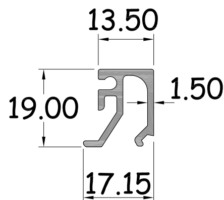
คิ้วในบานเพิ่มร่องกระจก 25.0 มิล รหัสสินค้า : 15176 WT. 0.276 Kg / M.
