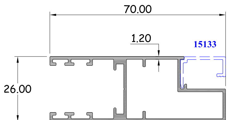
กรอบมุ้งนिरภัย รหัสสินค้า : 15132 WT. 0.717 Kg / M.
