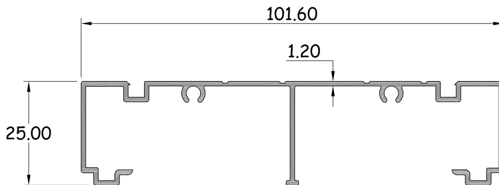
เฟรมข้าง รหัสสินค้า : 15104 WT. 0.701 Kg / M.
