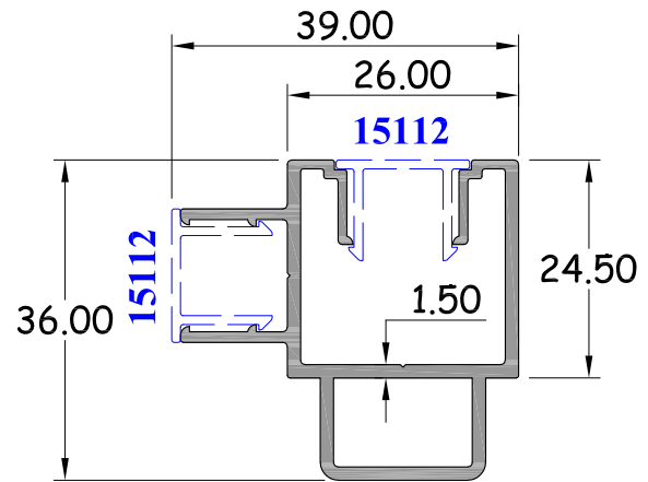
เสาเข็มมม 90 บานเลื่อน รหัสสินค้า : 15197 WT. 0.607 Kg / M.
