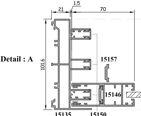
กรณีประกอบเฟรม 45 °
