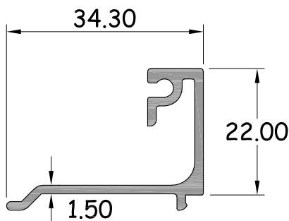
คิ้วกระจกห้อง 35 มิล หน้า 1.5 มิล รหัสสินค้า : 15180 WT. 0.340 Kg / M.
