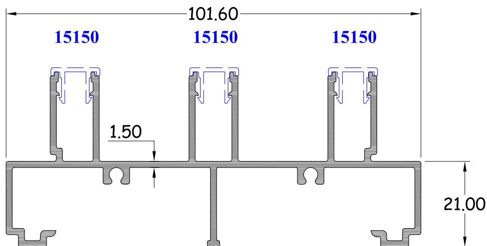
เฟรมข้าง+เฟรมบน 3 ร่อง หนา 1.5 มม รหัสสินค้า : 15162 WT. 1.405 Kg / M.
