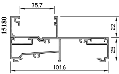
กรณีใส่กระจกมู๊ด
