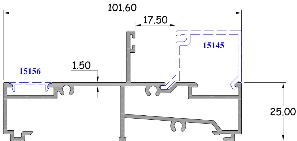
กล่องก้าน หนา 1.5 มิล (HOLLOW) รหัสสินค้า : 15155 WT. 1.305 Kg / M.
