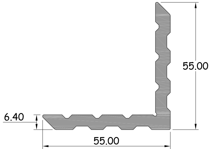
ฉากเข้ามุม บานเปิด,บานเพี้ยม รหัสสินค้า : 15187 WT. 1.488 Kg / M.
