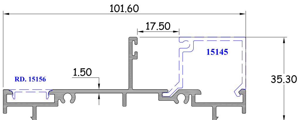
คาน C กรูฟ 2 ทาง หนา 1.5 มิล รหัสสินค้า : 15193 WT. 0.854 Kg / M.
