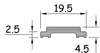
Transmission Rod รหัสสินค้า : 15157 WT. 0.145 Kg / M.
