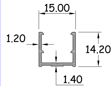
เดือยกุกญแ รหัสสินค้า : 15110 WT. 0.134 Kg / M.
