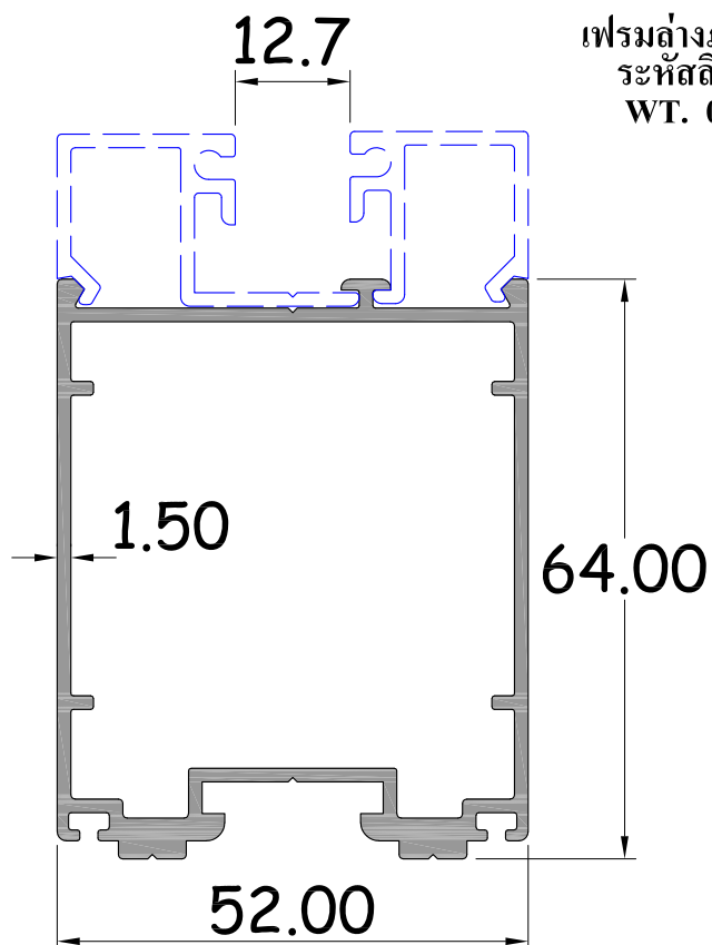
เสาบานเพี้ยม หน้า 1.5 มัด รหัสสินค้า : 15171 WT. 1.226 Kg / M.
