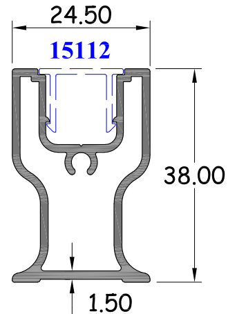
เสารับแรงบานเลื่อน(สตีฟไฟเนอร์) รหัสสินค้า : 15198 WT. 0.590 Kg / M.
