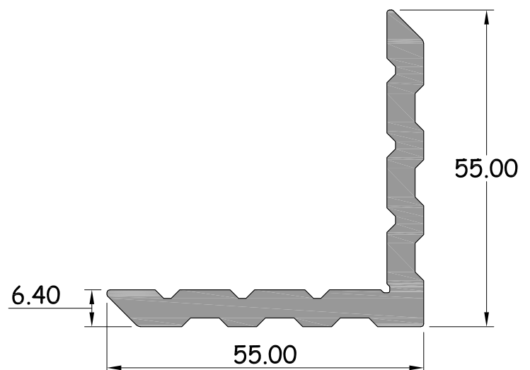
ฉากเข้ามุม บานเปิด,บานเพิ่ม รหัสสินค้า : 15187 WT. 1.488 Kg / M.
