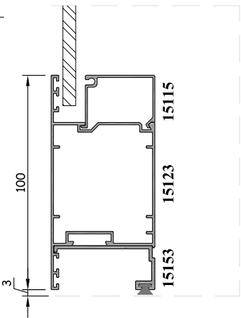
Detail : C กรณีทำภายใน
