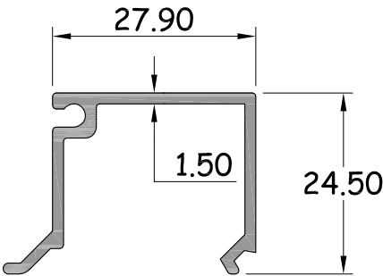
คิ้วตบกระຈก หนา 1.5 มิล รหัสสินค้า : 15145 WT. 0.356 Kg / M.
