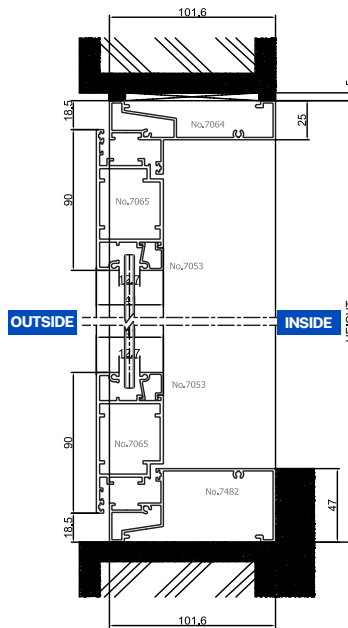
Section Double Door
