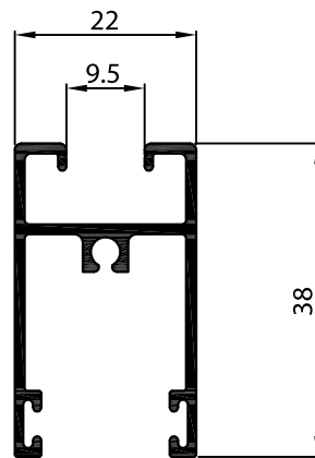
P-126778 ขวงบน-ล่าง (ล้อตลับและล้อเล็กพิเศษ)
