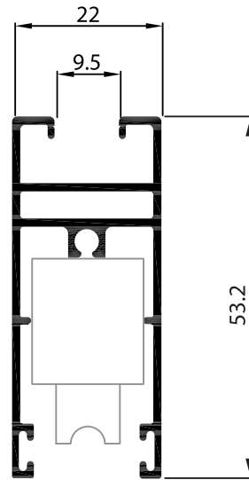
P-123167 ขวงบน-ล่าง (ล้อตลับร่อนยู) *มี Hollow ป้องกันสกรูโดนกระชากแตก*
