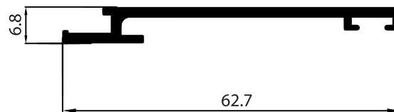
P-203878 ฟ้ापี้ดรางแขวน
