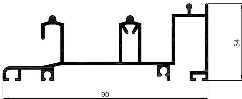
P-126799 เฟรม บน-ล่าง 9 ซม. (กรณีเตี้ย)
