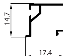
P-093873 ค้ิ้วบานแขวน-ส่วิง
