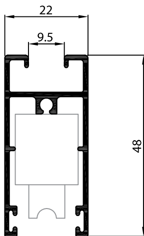
P-126777 ขวงบน-ล่าง (ล้อตลับร่อนยู)
