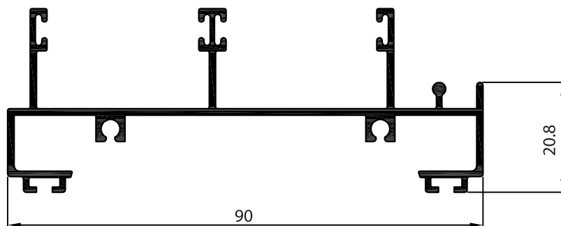
P-126801 เฟรมข้าง 9 ซม.
