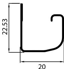
P-103088 ก้านตก (ใช้ร่วมกับเฟรมล่าง = ก้านตก) (ใช้ร่วมกับเฟรมบน = ก้านสอด)
